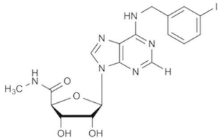
IB-MECA
